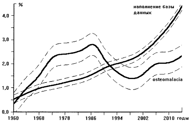
Рис. 1. Результаты математического статистического моделирования динамики наполнения публикациями из рецензируемых журналов базы данных «Medline» и количества публикаций на ключевое слово «Osteomalacia». Обозначения: по вертикальной оси – доля (в %) ежегодно включаемых в базу данных публикаций к общей массе статей по проблеме, по горизонтальной оси – годы; сплошная линия – тренд изменения показателя, аппроксимация сплайнами с параметрами модели P=0,1 ( p=0,05 ); пунктирная линия – полуширина доверительной полосы (1,96 \sigma )
