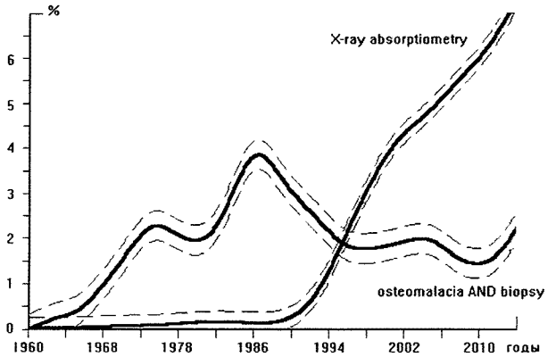
Рис. 2. Результаты математического статистического моделирования ежегодного прироста количества публикаций в рецензируемых журналах в базе данных количества на ключевые слова «Osteomalacia AND biopsy» и «X-ray absorptiometry». Обозначения: по вертикальной оси – доля (в %) ежегодно включаемых в базу данных публикаций к общей массе статей по проблеме, по горизонтальной оси – годы; сплошная линия – тренд изменения показателя, аппроксимация сплайнами с параметрами модели P=0,1 ( p=0,05 ); пунктирная линия – полуширина доверительной полосы (1,96 \sigma )
