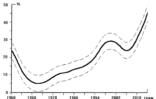
Рис. 3. Результаты математического статистического моделирования ежегодной доли публикаций на ключевое слово «Osteomalacia AND Case report». Обозначения: по вертикальной оси – доля (в %) статей на ключевые слова «Osteomalacia AND Case report» от общего количества статей по проблеме остеомалиции, опубликованных за год, по горизонтальной оси – годы; сплошная линия – тренд изменения показателя, аппроксимация сплайнами с параметрами модели P=0,1 ( p=0,05 ); пунктирная линия – полуширина доверительной полосы (1,96 \sigma )
